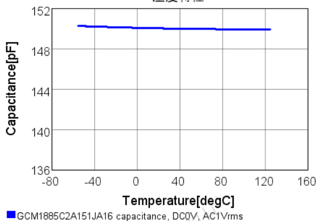
温度特性
