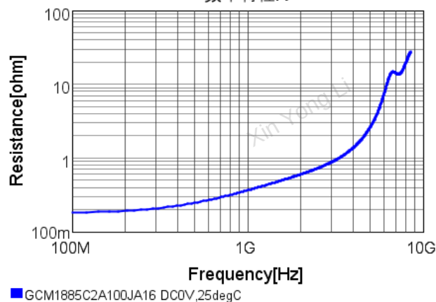
频率特性R
