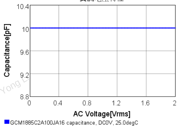
交流电压特性
