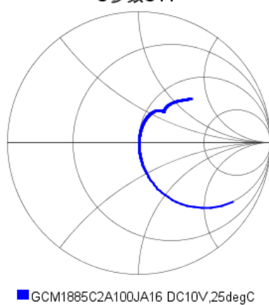
S参数S11
