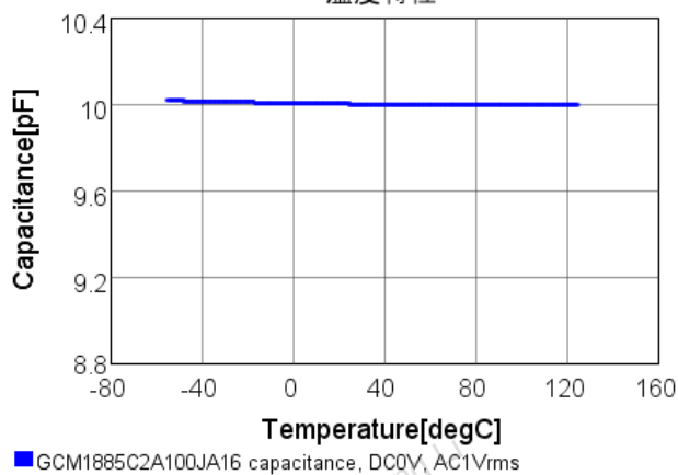
温度特性
